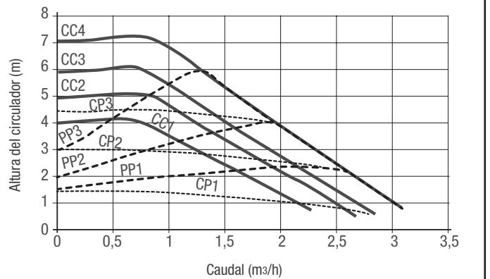
Altura residual disponible para el sistema de BAJA TEMPERATURA
