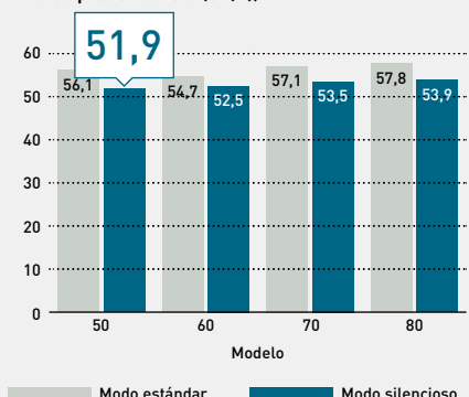
Nivel de presión sonora (dB(A)).
