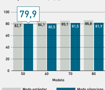
Nivel de potencia sonora (dB(A)).
